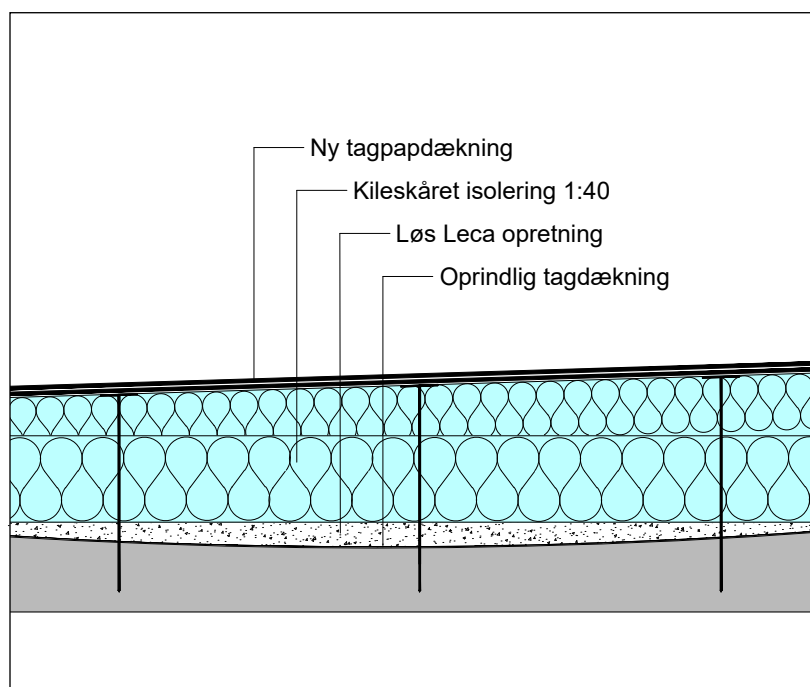
Figur 8.1: Underlag for renovering oprettet med løs Leca.
