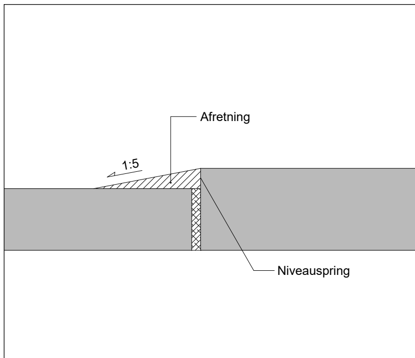
Figur 4.1: Opretning af spring i underlag
