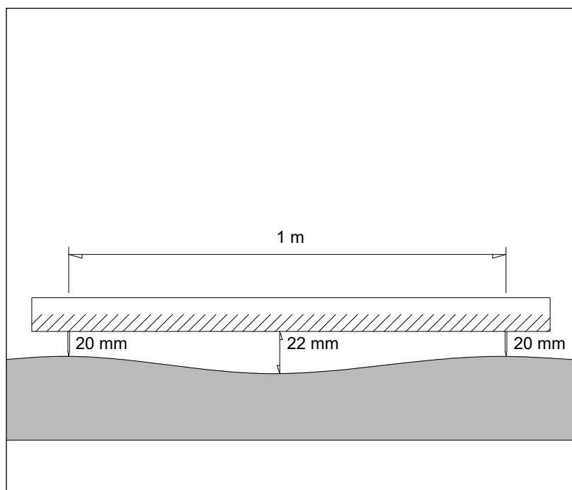
Figur 9.2: Måling af lunke i underlag.
