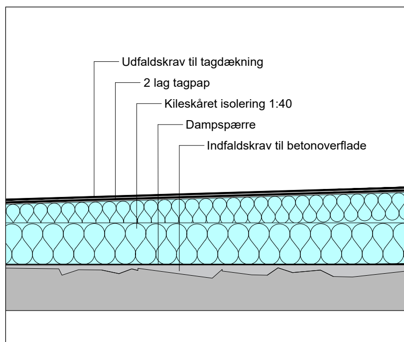
Figur 1.2.1.: Udfaldskrav til tagdækning og indfaldskrav til underlag.
