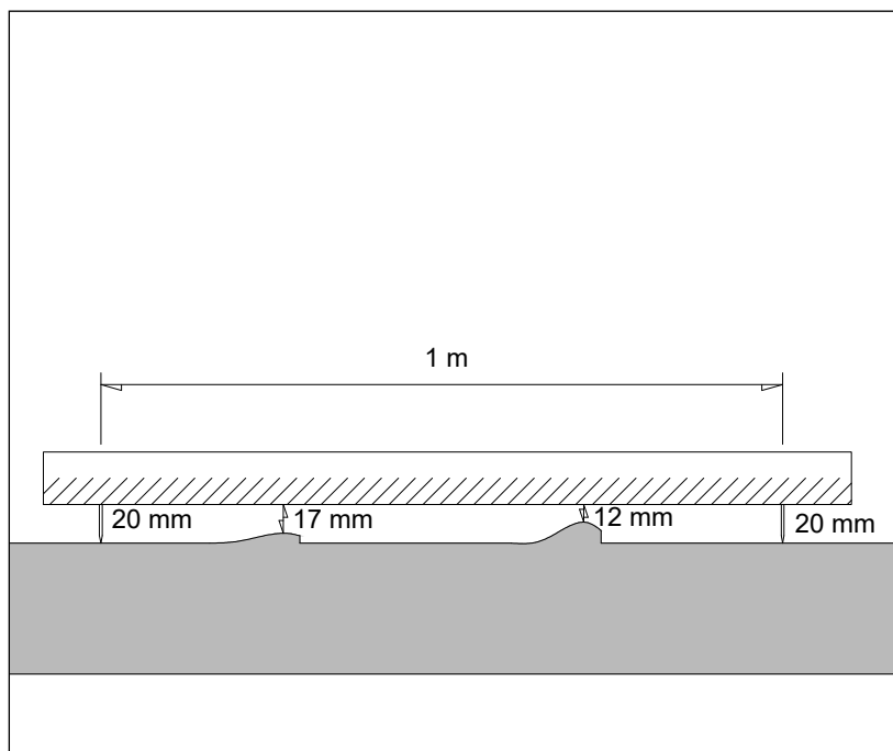
Figur 9.3: Måling af grater.
