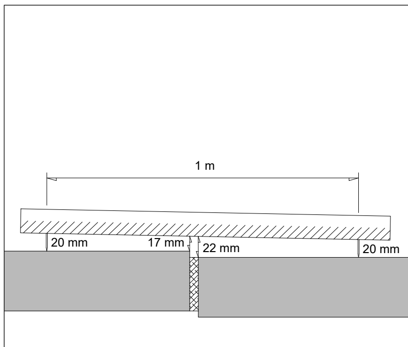
Figur 9.4: Måling af spring.
