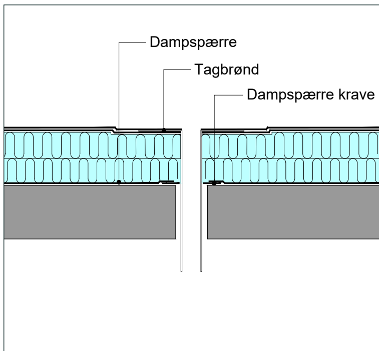
Figur 4.4.4: Tætning ved tagbrønd. Kan eventuelt udføres med dampspærrekrave.
