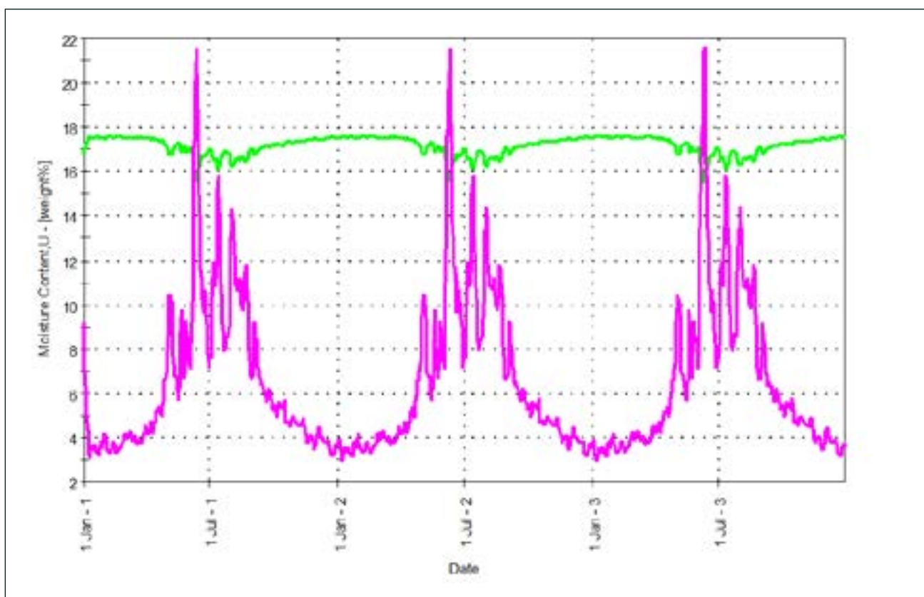
Figur 3.9.1: Simulering af fugtforholdene i et uventileret tagelement med 300 mm mineraluldisolering og hvor fugt er spærret inde mellem en diffusionstæt dampspærre og en tæt tagpapdækning. Grøn kurve viser fugtindholdet i krydsfineren og lilla viser kontrollaget, som et fiktivt meget tyndt lag filt placeret i bunden af tagkonstruktionen til vurdering af fugtvandring gennem året.
