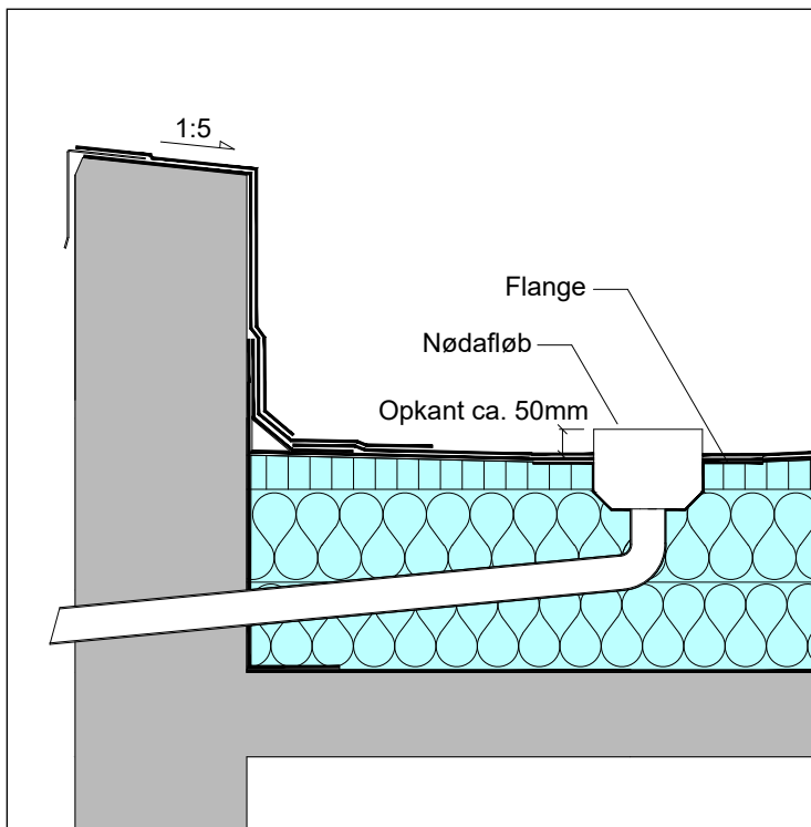
Figur 2.1.6.2: Indvendigt nødafløb med hævet afløbsskål.
