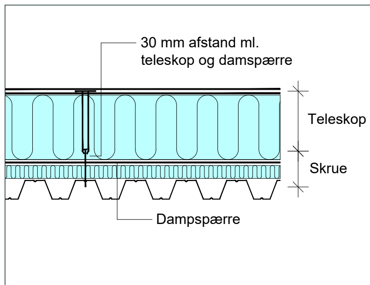
Figur 4.4.1: Valg af beslag ved oprykket dampspærre på underlag af profilerede stålblader.
