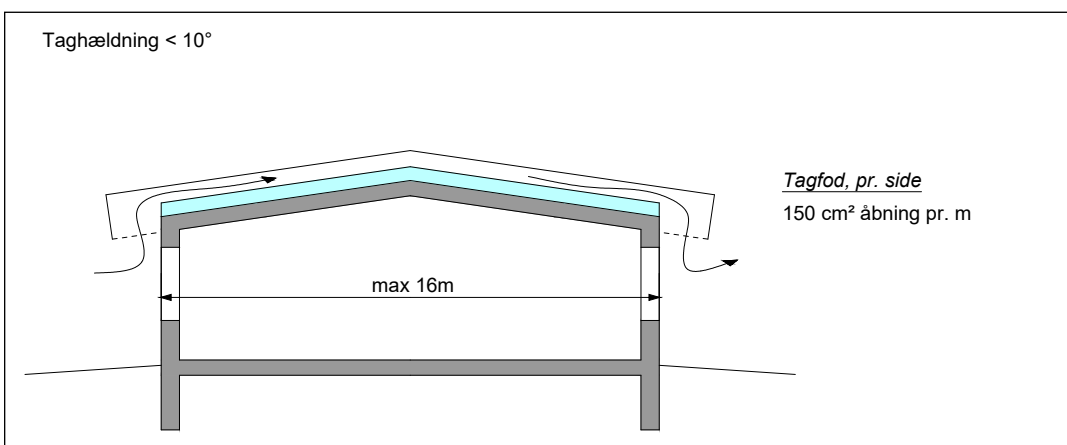
Figur 3.6.1.4: Nettoareal af ventilationsåbninger ved tagfod ved taghældning <math>< 10^\circ</math>.
