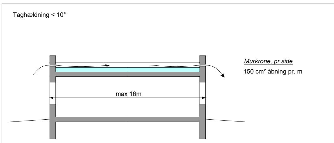
Figur 3.6.1.3: Nettoareal af ventilationsåbninger i murkrone ved taghældning <math>< 10^\circ</math>.
