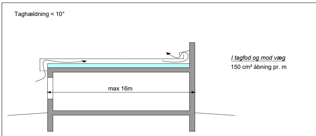
Figur 3.6.1.2: Nettoareal af ventilationsåbninger ved tagkanter og mur ved taghældning <math>< 10^\circ</math>.
