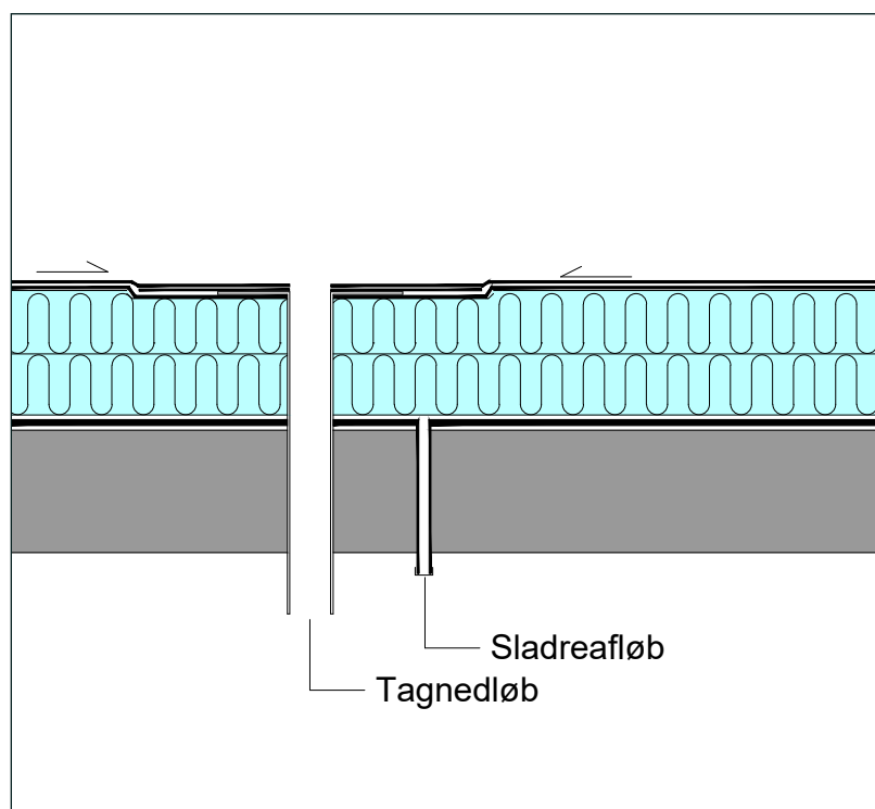
Figur 3.2.6.1.2: Sladre afløb.
