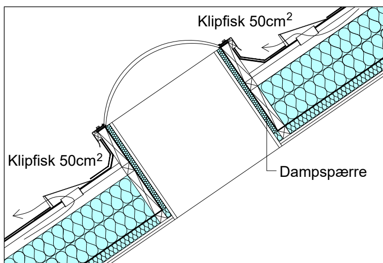
Figur 3.6.5.2: Udskramning eller klipfisk ved tage med hældning over 10^\circ .
