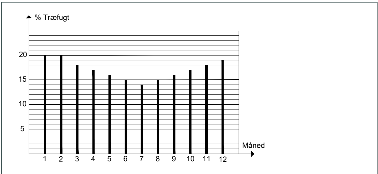
Figur 3.8.1.2: Årsvariation af forventet maksimal træfugt i ventilerede tagkonstruktioner i ligevægt med udeluften.
