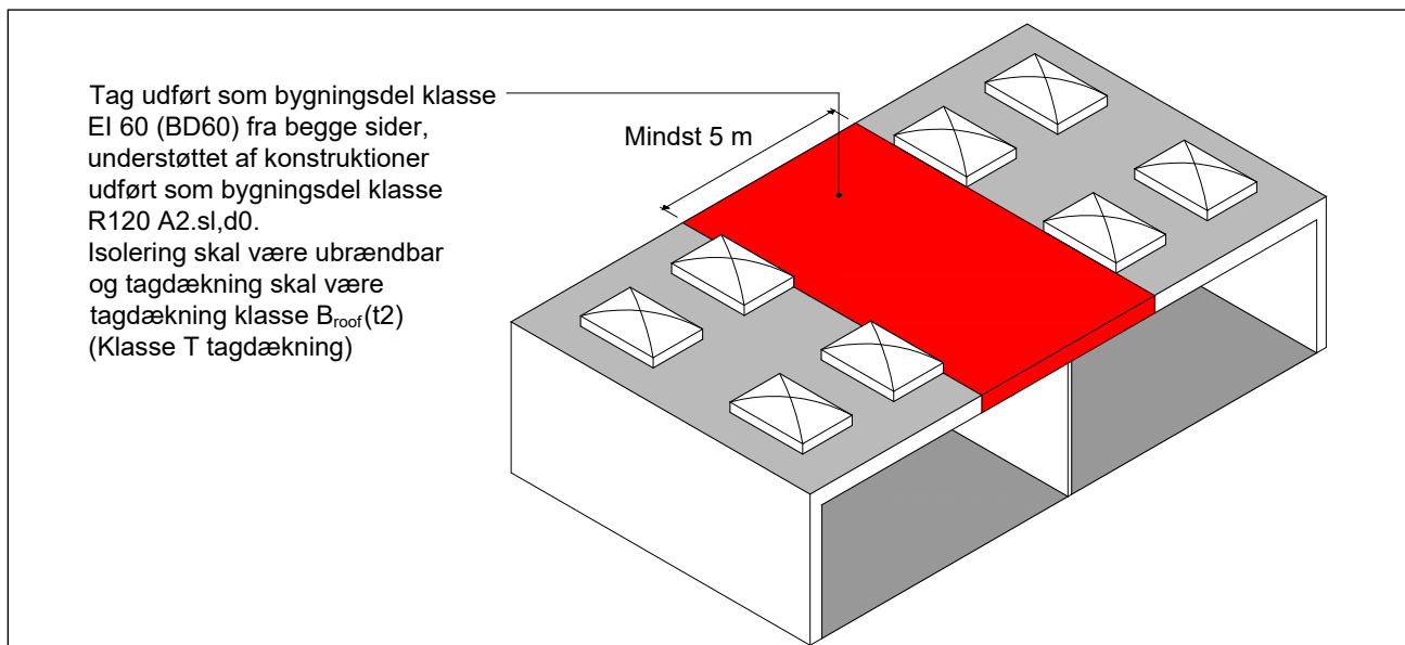
Figur 8: Brandkamserstatning ved sektionstvæg i industri- og lagerbygninger.
