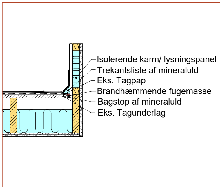
Figur 31: Ved udskiftning eller montering af nye ovenlys uden merisolering lukkes fugen mellem ovenlys og den eksisterende tagdækning med en blød mineraluldsstopning og et brandteknisk egnet fugemateriale. En trekantsliste lægges i det bløde fugemateriale.
