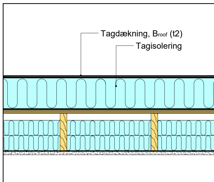
Figur 21: Klasse B_{\text{roof}} (t2) tagdækninger på underlag af isolering, klasse F eller højere kan anvendes til bygninger omfattet af BR18. Hvis der anvendes tagisolering af B-s1, d0 (klasse A) kan tagdækningen også anvendes til bygninger omfattet af de Tekniske Forskrifter.
