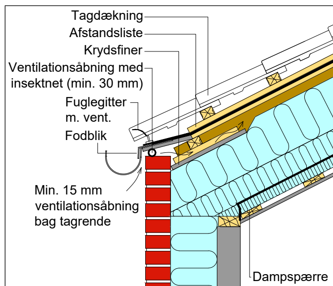
Figur 12.1.4.1 Tagfod uden udhæng. Der skal være jævnt fordelte ventilationsåbninger ved tagfod til at sikre tilstrækkelig ventilation. Anvendes insektnet i ventilationsåbninger, skal arealet fordobles
