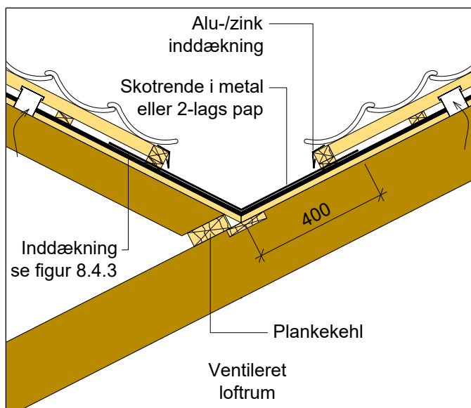
Figur 12.4.2 Skotrende med plankekehl - vandret snit. Detalje ved tilslutning til skotrende ses på figur 12.4.3.
