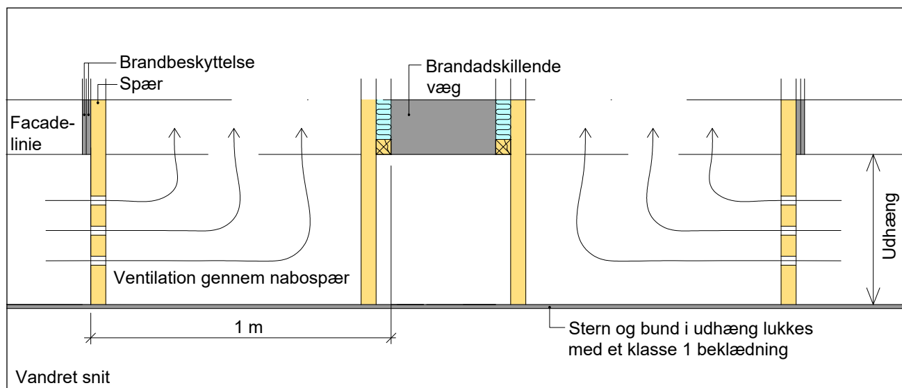
Figur 10.3.3 Brandkamserstatning EI 60 (BD-bygningsdel 60) 1,0 m på hver side af brandsektionsvæg i tagrum.
