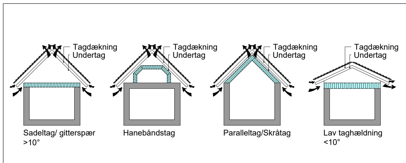
Figur 4.1.1 Princip for ventilation af undertag. Se også PTM-anvisning nr. 4 Fugt.
