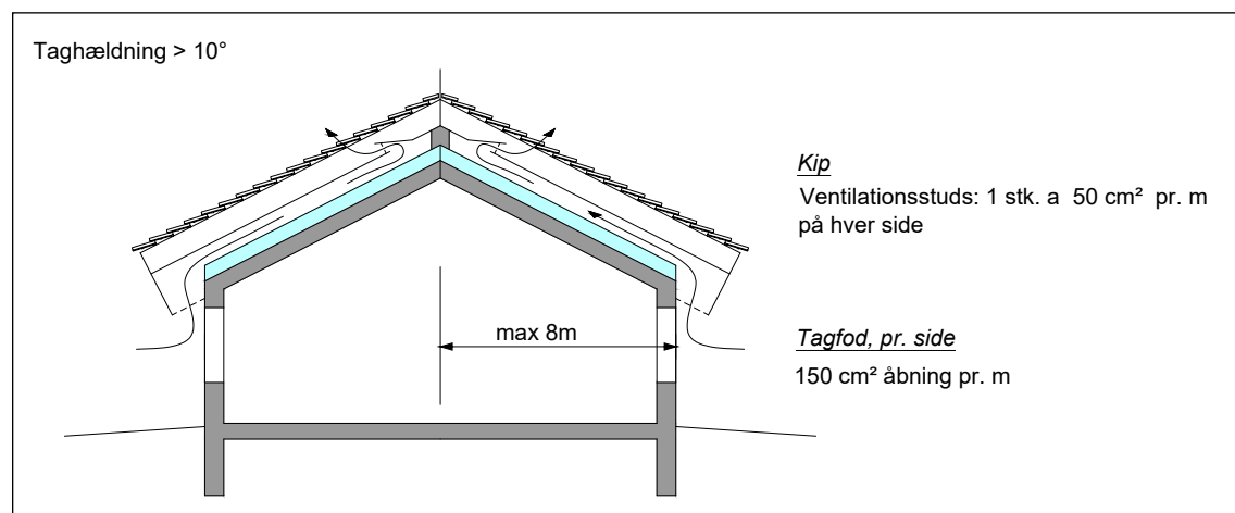
Figur 4.1.2.1 Dimension/areal af ventilationsåbninger ved ventilation af paralleltag/skråtag fra tagfod til hver side af tagkip ved taghældning >10°
