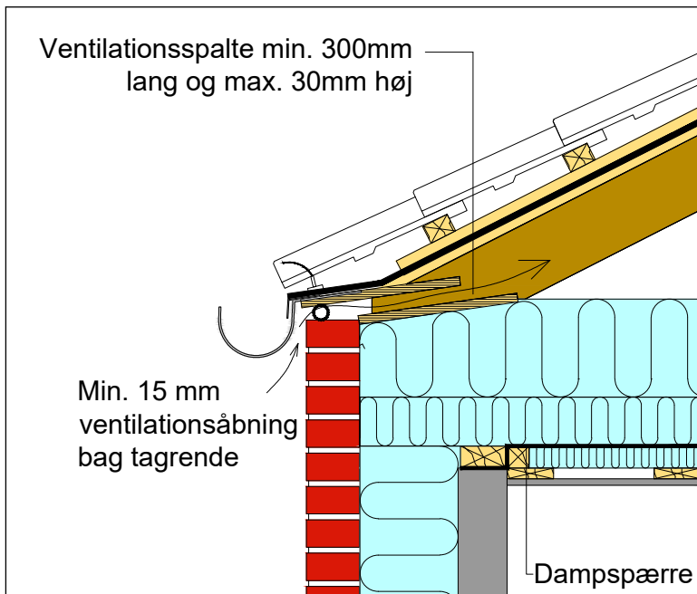
Figur 10.1.1 Tagfod uden udhæng ved konstruktion med loftrum udført med brandsikker ventilationsåbning.
