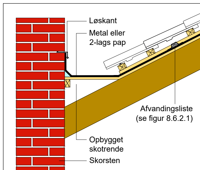
Figur 12.4.2.1 Skotrende bag skorsten. Skotrende opbygges så den får fald fra midten af skorsten og ud mod siderne. Skotrenden udføres med to lag tagpap på opbygget underlag. Skotrenden er forsynet med overpap eller en zink-/aluinddækning.
