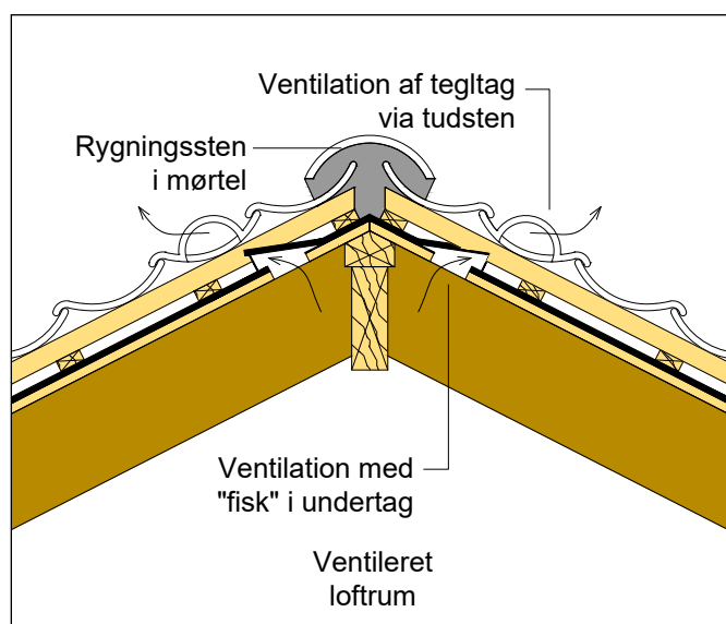
Figur 12.3.1.2 Grat på tag med mørtel i rygning - vandret snit. Ventilationen over undertaget udføres med tudsten placeret langs gratrygning. Ventilation, her vist med studs, monteres i undertag mellem hvert spærfag i gratkonstruktionen.
