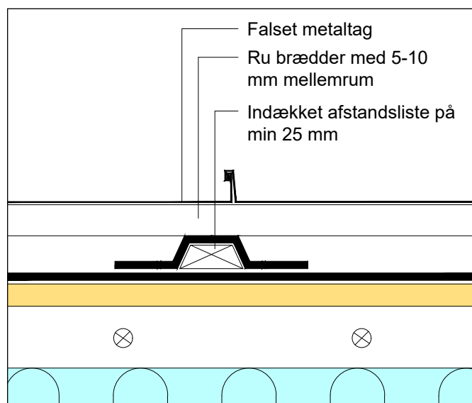
Figur 11.2.3 Falsed metaltag udlagt på bræddeunderlag over fast undertag med inddækkede afstandslister.
