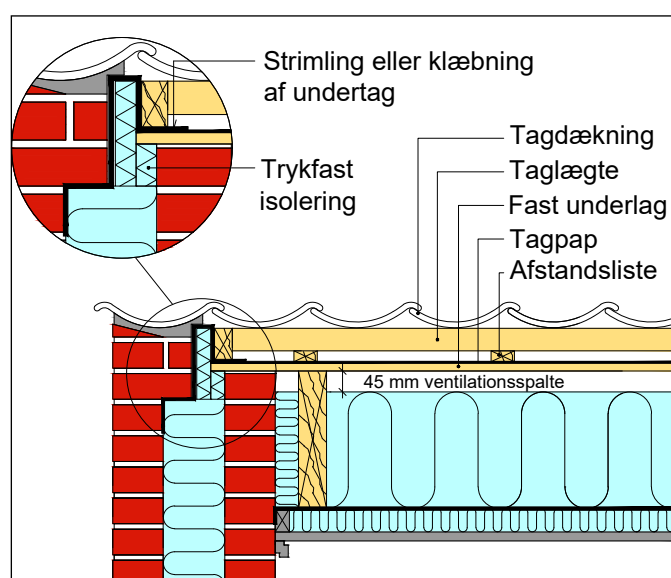
Figur 12.5.1.1 Gavl uden udhæng. Det skal sikres, at vand kan ledes effektivt væk og ikke ind i ydervæggen.
