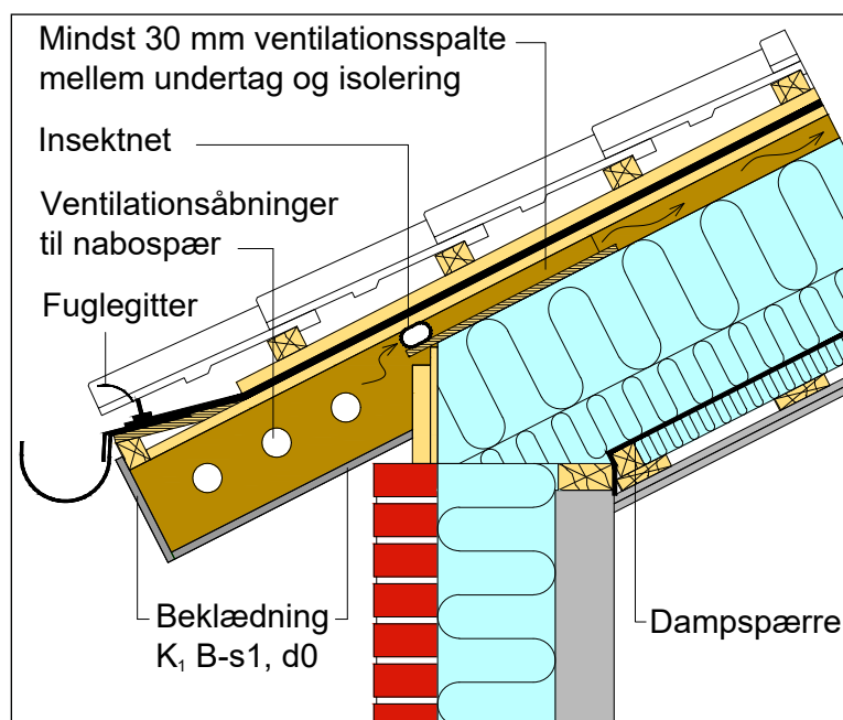
Figur 10.2.1 Tagfod med udhæng. Brandkrav til ventilationsspalte samt beklædning 1 m til hver side af brandkamserstatning. Dette er et krav i Bygningsreglementer og gælder for rækkehuse og etageejendomme
