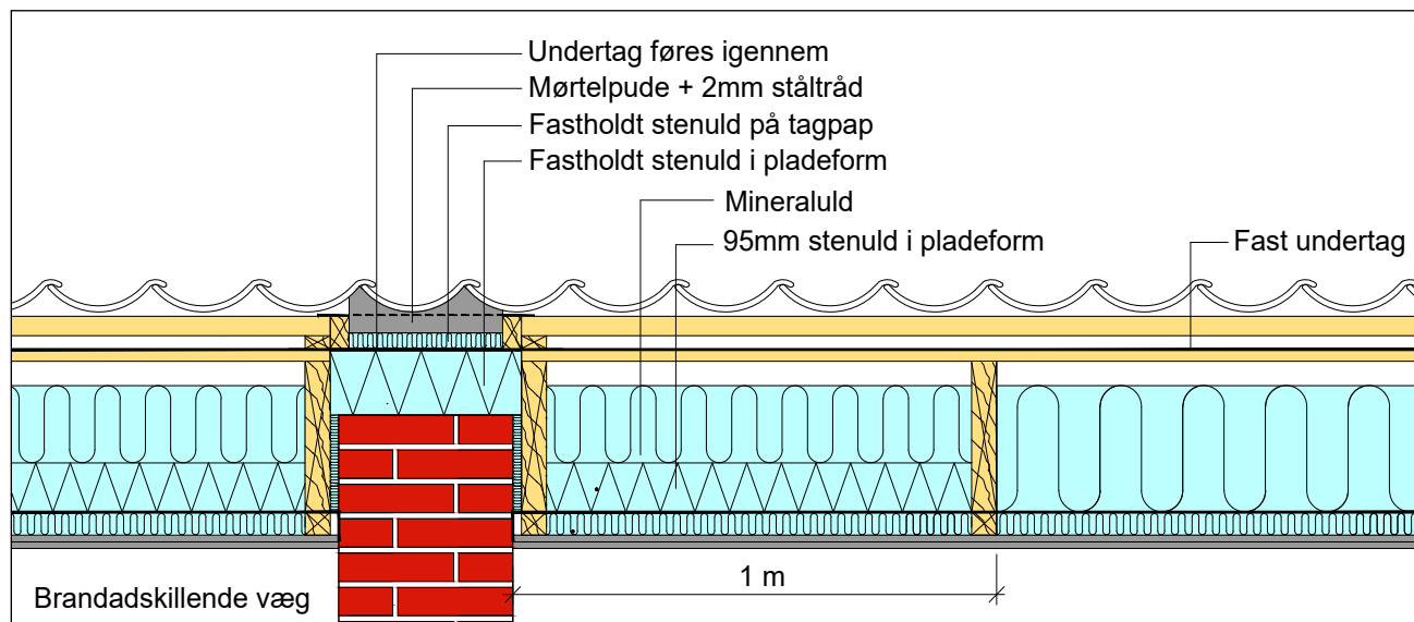
Figur 10.3.4. Brandkamserstatning udført på begge sider af en brandadskillende væg, lukkes tæt til undersiden af tagdækningen med mørtel på tyndt underlag af fastholdt stenuld
