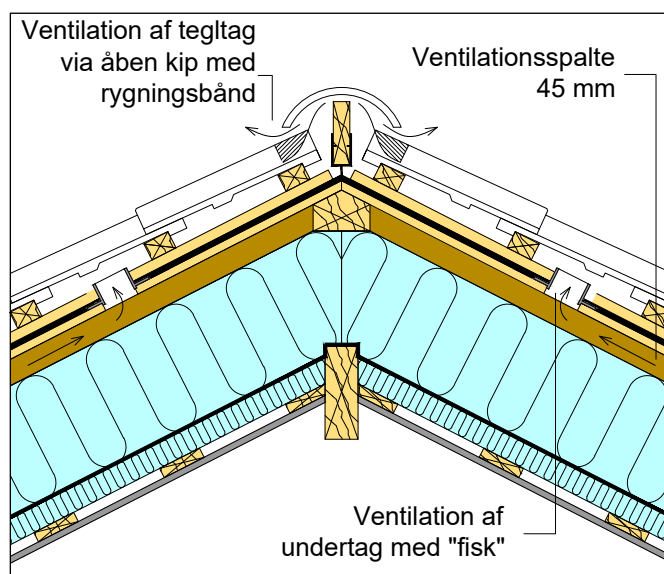
Figur 12.2.2.1: Kip i paralleltag med undertag ventileret med studs på hver side af rygning. Ventilation mellem tagsten og undertaget sker her gennem den åbne kip.
