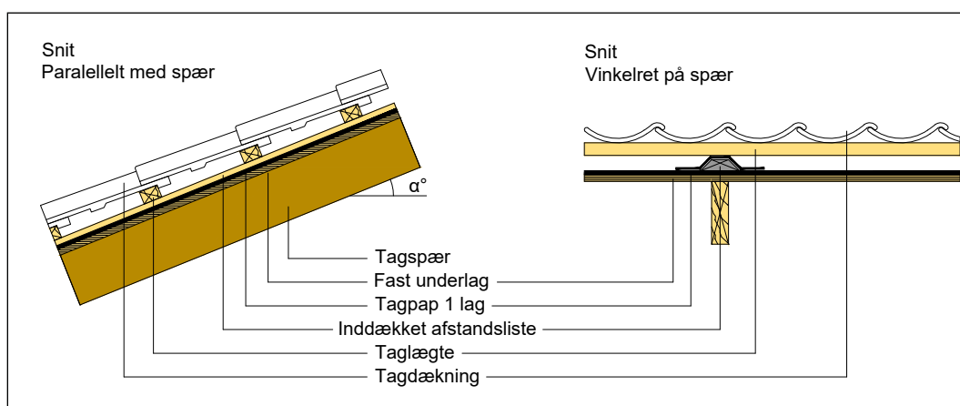
Figur 9.2 Tag med forholdsvis lav hældning ( 25^\circ > \alpha \geq 11,1^\circ ) og åben tagdækning. Der anvendes et lag tagpap. Afstandslister er affasede, uimprægnerede og inddækkede.
