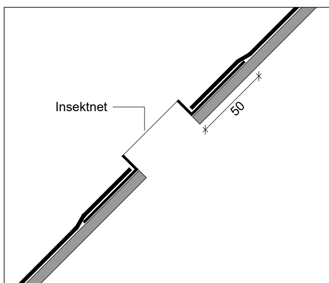
Figur 4.1 Ventilationsstudse med flange til klæbning af tagpap
