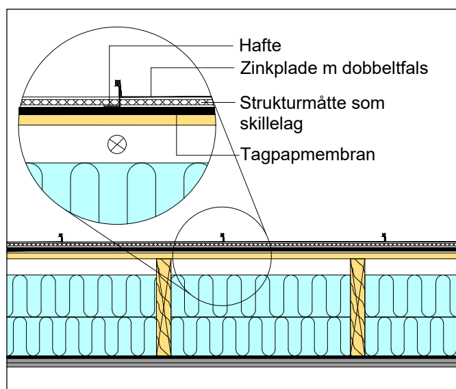
Figur 11.2.2 Zinkplade med dobbeltfals og strukturmåtte som skillelag
