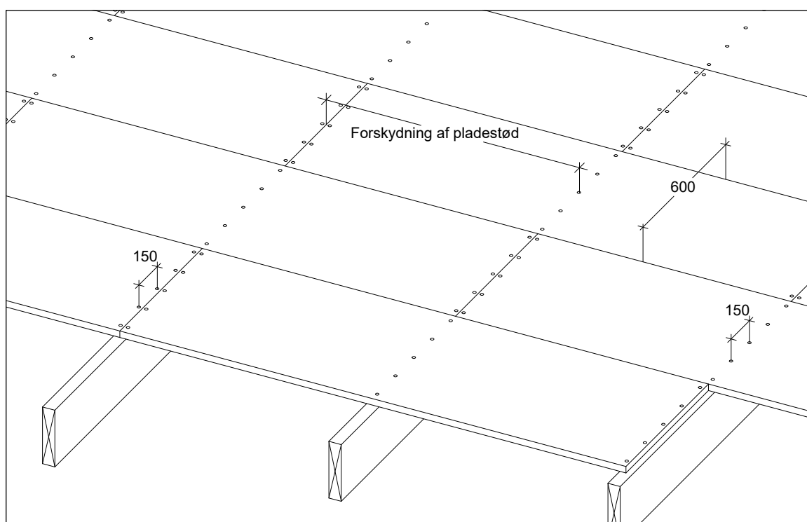
Figur 3.2.1.2 Oplægningsmønster for 15 mm krydsfinerplader med pladedimension 0,61 x 2,44 m
