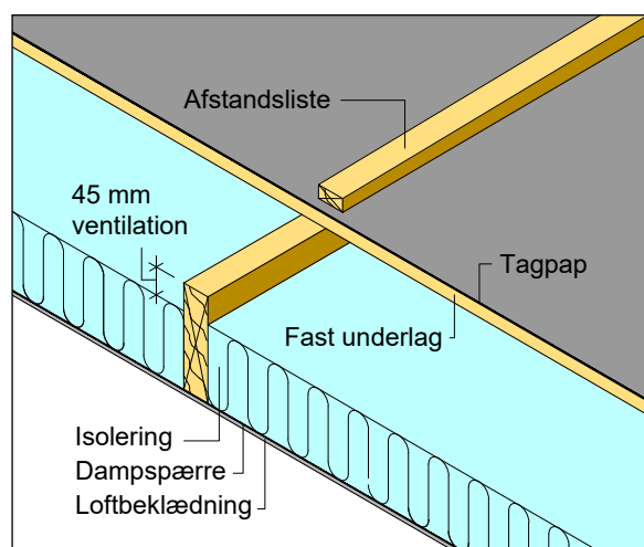
Figur 9.5 Paralleltag med stor hældning og et lag tagpap. Afstandslist er trykimprægnerede og inddækkes ikke.
