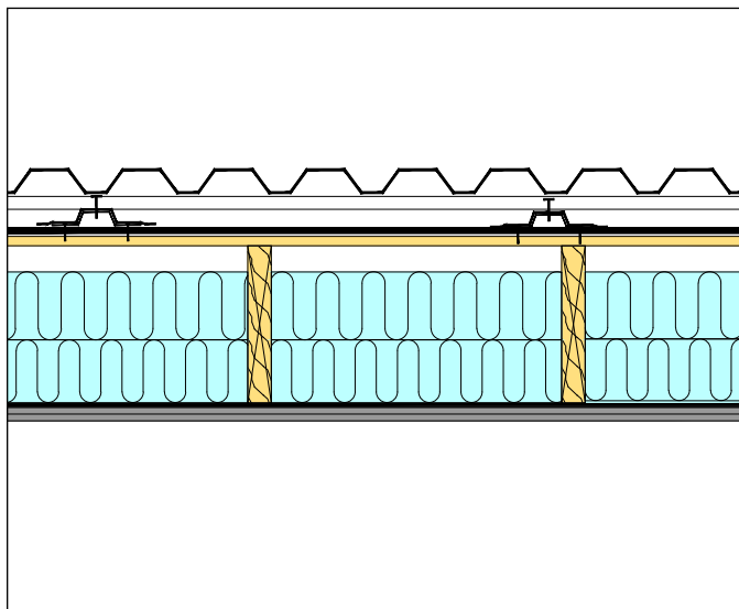
Figur 11.1.1 Stålpladedækning hævet op på lægtesystem
