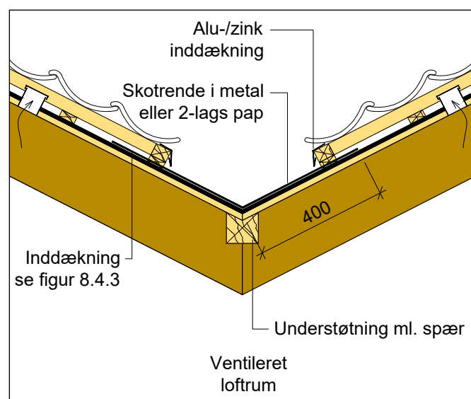
Figur 12.4.1 Skotrende - vandret snit. Er skotrenden ikke udført med kehlplanke eller kehlspær, etableres understøtning af skotrendens bund som vist. Detalje ved tilslutning til skotrende ses på figur 12.4.3.
