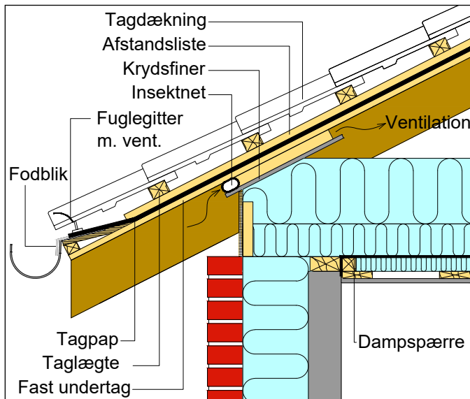
Figur 12.1.1.1 Tagfod med udhæng. Der skal være jævnt fordelte ventilationsåbninger ved tagfod til at sikre tilstrækkelig ventilation. Anvendes insektnet i ventilationsåbningen, skal arealet fordobles til 30 mm.
