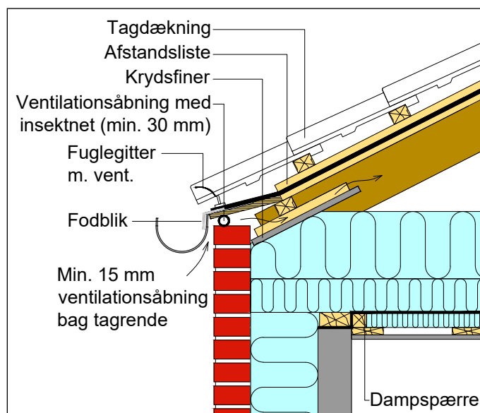
Figur 12.1.2.1 Tagfod uden udhæng. Der skal være jævnt fordelte ventilationsåbninger ved tagfod til at sikre tilstrækkelig ventilation. Anvendes insektnet i ventilationsåbningen, skal arealet mindst fordobles. Undtagelsesvis ved skotrender kan det være nødvendig at ventilere med ventilationsstudser i begge ender af spærfaget.
