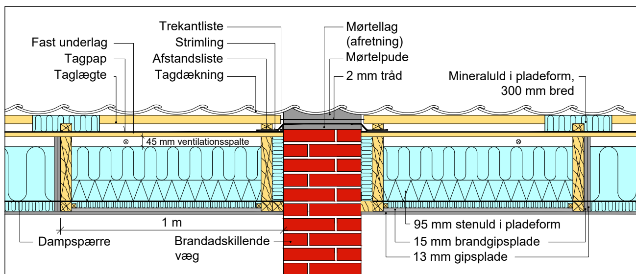
Figur 10.3.2 Brandkamserstatning ved paralleltage. EI 60 (BD-bygningsdel 60) konstruktion
