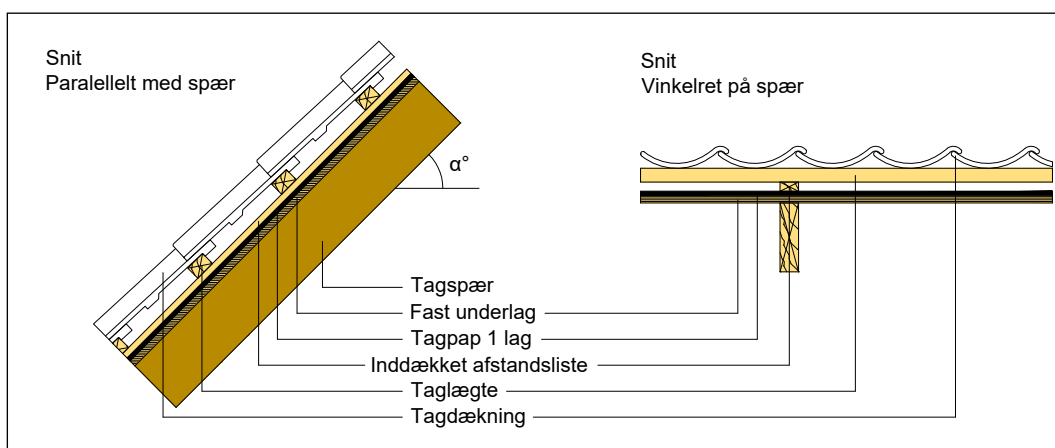
Figur 9.1 Tag med stor hældning ( \alpha > 25^\circ ). Der anvendes et lag tagpap. Afstandslister er trykimprægnerede, skarpkantede og inddækkes ikke. Hvis underlaget er ujævnt, f.eks. i forbindelse med renovering af gammelt undertag på brædder, bør afstandslisterne lægges i asfaltklæber.
