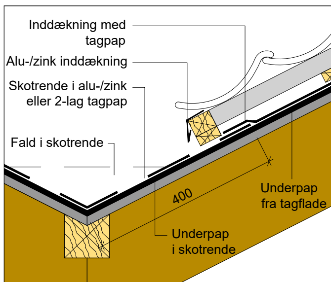
Figur 12.4.3 Detalje af inddækningsprincip i skotrende - vandret snit. Alu-/zinkrende kan alternativt udføres som overpap.
