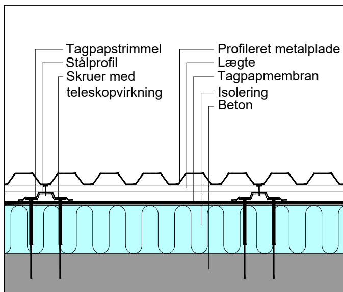
Figur 11.1.3 Metalpladedækning hævet op på lægtesystem. (Uventileret, varmt tag)
