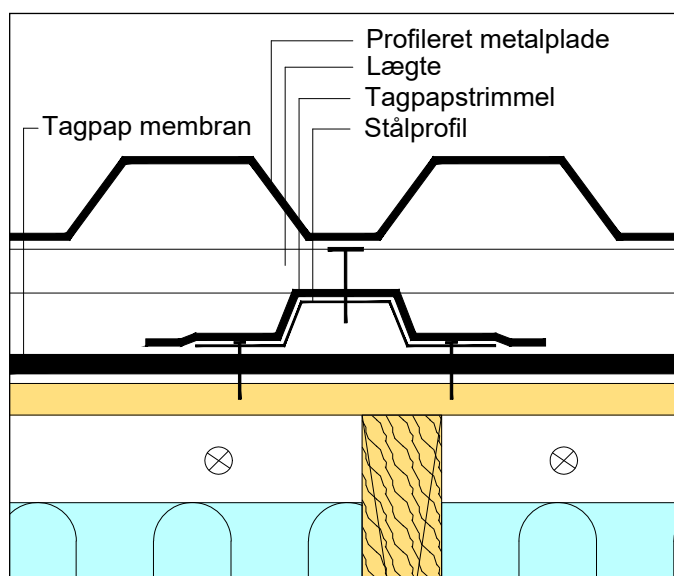
Figur 11.1.2 Metalpladedækning hævet op på lægtesystem - detalje. (Ventileret, koldt tag) og stålprofil lukkes med tagpap øverst
