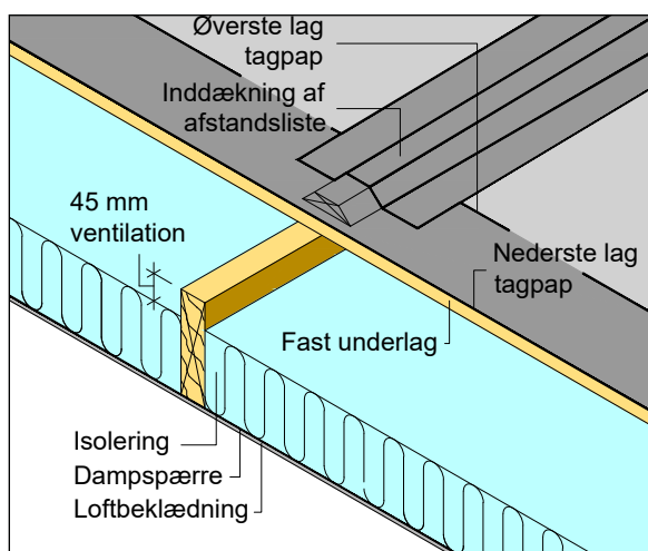
Figur 9.4 Paralleltag med lav hældning og åben tagdækning. Der anvendes to lag tagpap og inddækkede afstandslist. Endvidere vises den generelle konstruktionsopbygning for et paralleltag med ventilationshulrum
