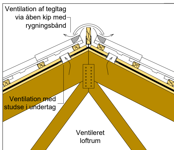
Figur 12.2.1.2 Kip med udluftning af undertaget med ventilationsstuds anbragt nær kip. Tagpap føres hen over kip, og rygningsplanken fastgøres med kipbeslag. Ventilation mellem tagsten og undertaget sker her gennem den åbne kip.
