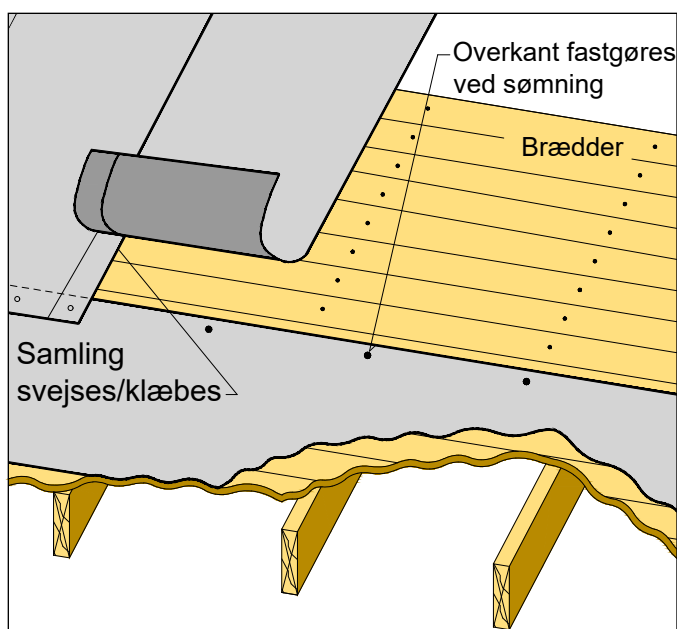
Figur 7.1.1.1 Tagpapbaner sømmes til bræddeunderlag (eller plader) parallelt med eller vinkelret på tagets faldretning. Fastgørelse til underlaget sker pr. 150-200 mm og 2 cm fra kanten. For at forhindre at vindsug under byggeperioden river tagpappen løs, monteres afstandslisters i takt med udlægning af tagpap
