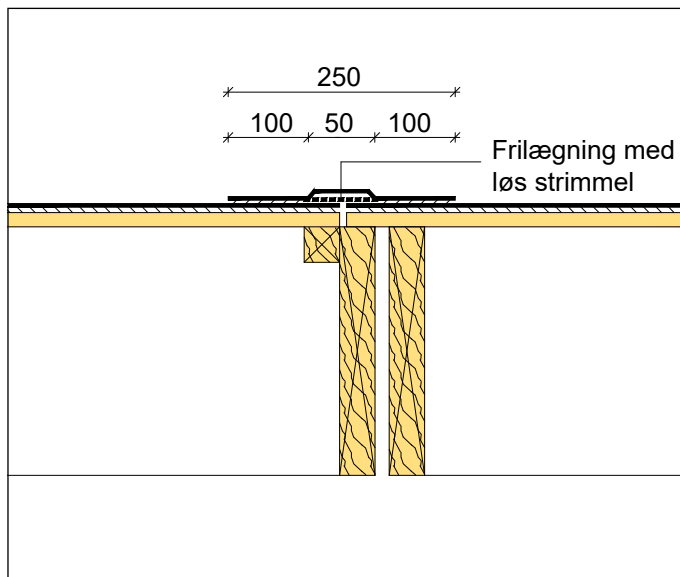
Figur 7.3.1.2 Strimling af elementsamling med frilægning. Anvendes PTM DuraFlex (PF 3500 SBS) til strimling kan frilægning udelades
