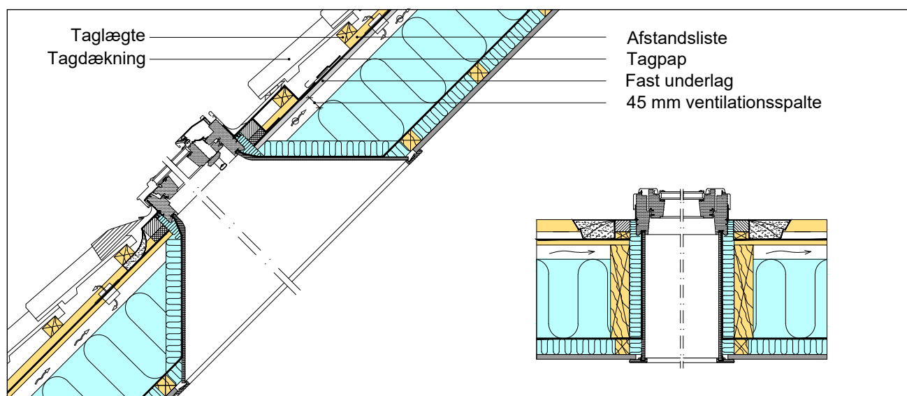
Figur 12.6.3.1 Tilslutning til ovenlys. Vand skal ledes effektivt uden om ovenlys, både i plan med tagdækningen og undertag.
