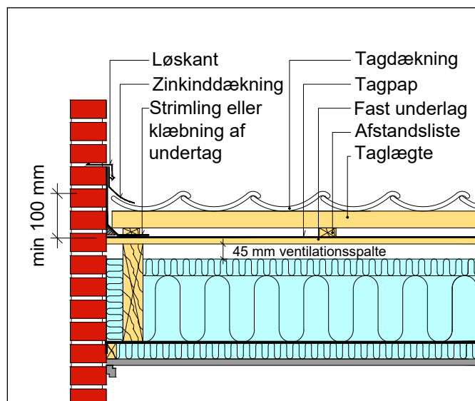
Figur 12.4.3.1 Tilslutning mod mur. Inddækningshøjde min. 100 mm.
