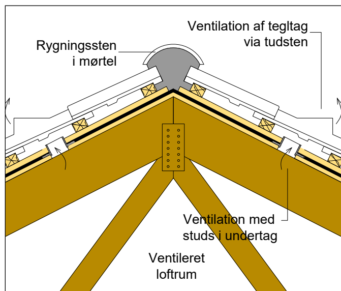
Figur 12.2.1.1 Kip med udluftning af undertaget gennem ventilationsstuds på hver side af rygning. Der skal etableres tilstrækkelig og jævnt fordelt ventilation af undertaget. Da rygning er udført i mørtel, skal der ved falstagsten også etableres ventilation af hulrummet mellem tagsten og undertaget, her vist med tudsten.
