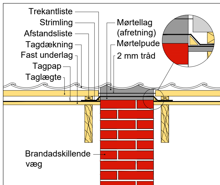
Figur 10.3.1 Brandadskillelse mellem åbne tagrum
