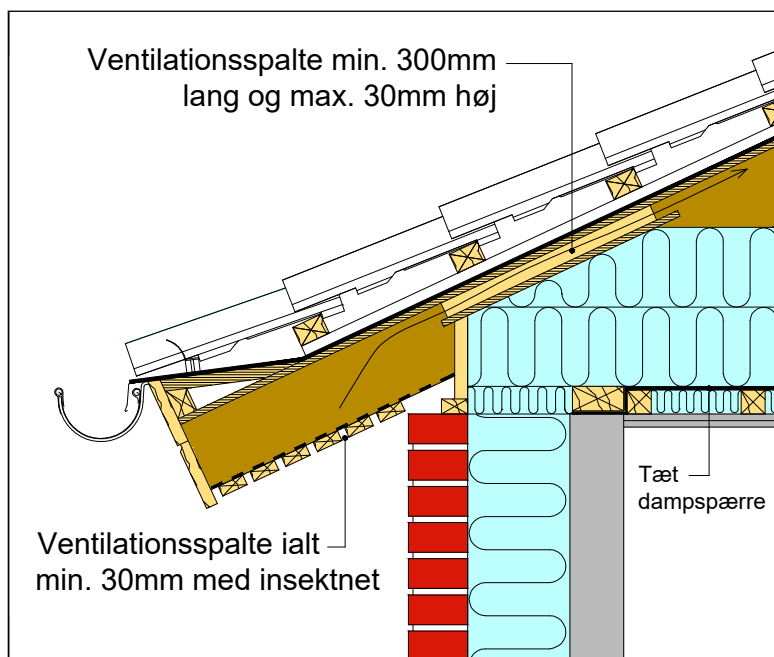
Figur 10.1.2 Tagfod med udhæng ved konstruktion med loftrum udført med brandsikker ventilationsåbning.
