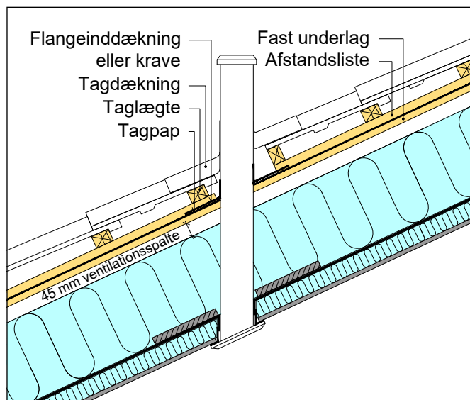
Figur 12.6.1.1 Rørgennemføring med ind-dækninger i niveau med både tagdækning og undertag, samt tæt dampspærre på konstruktionens underside.
