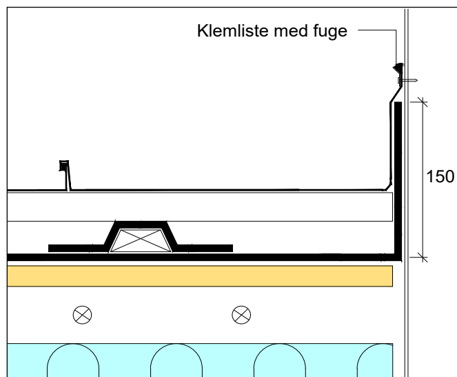
Figur 11.3.1 Inddækning af gennemføring ved falset metaltag på underlag af brædder
