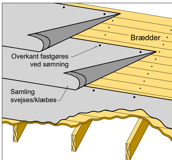
Figur 7.1.1.2 Tagpapbaner kan også fastgøres vinkelret på tagets faldretning
