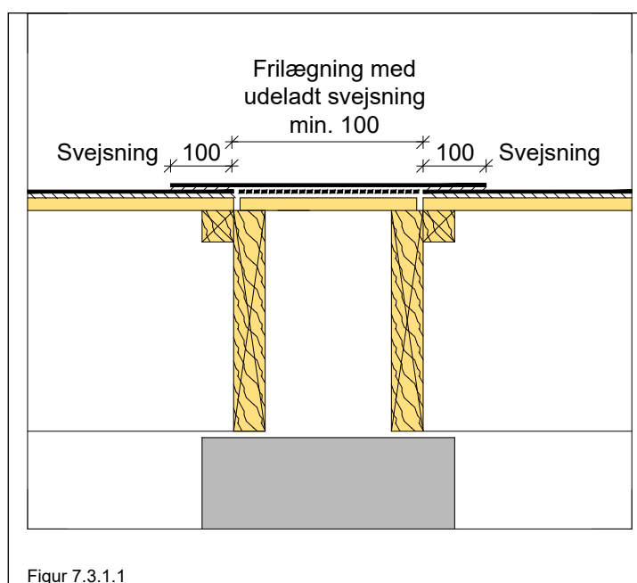
Figur 7.3.1.1 Strimling af elementsamling ved endesamling med tilpasningsstykke. Anvendes PTM DuraFlex (PF 3500 SBS) til strimling kan frilægning udelades
