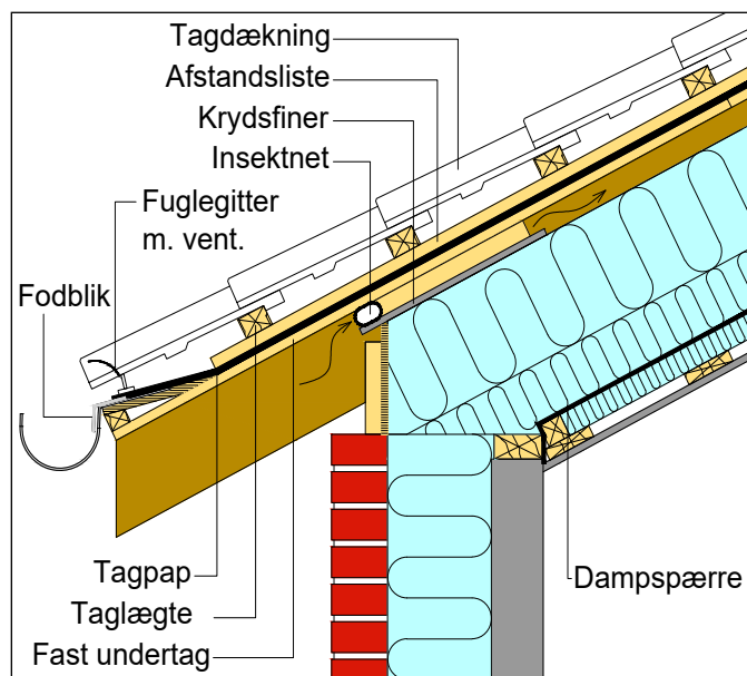
Figur 12.1.3.1 Tagfod med udhæng. Der skal være jævnt fordelte ventilationsåbninger ved tagfod til at sikre tilstrækkelig ventilation. Anvendes insektnet i ventilationsåbningen, skal arealet fordobles
