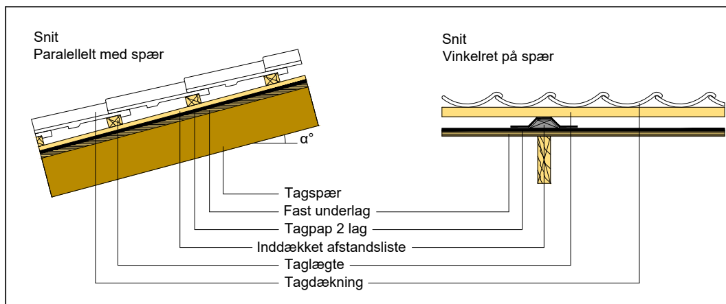
Figur 9.3 Tag med lav hældning ( 11,1^\circ > \alpha \geq 1,5^\circ ) og åben tagdækning. Der anvendes to lag tagpap. Afstandslisterne er affasede, uimprægnerede og inddækkede med et lag tagpap
