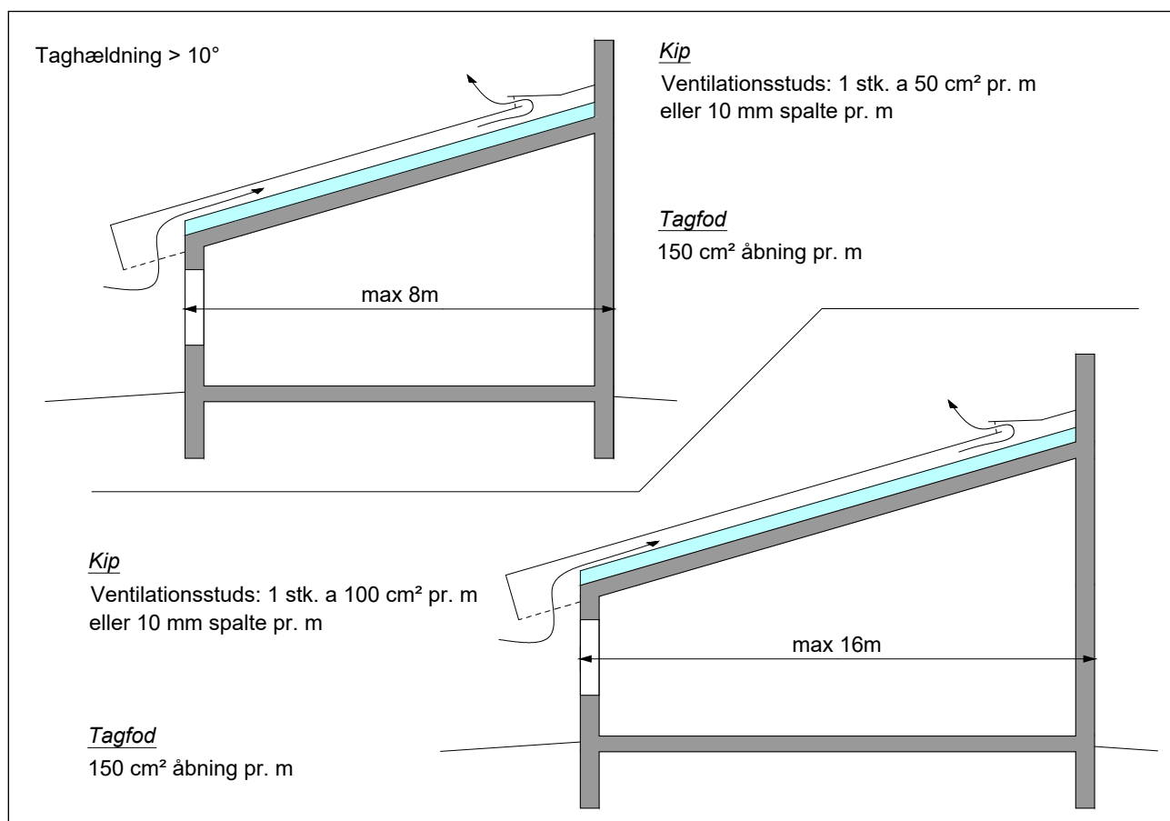
Figur 3.6.1.9: Nettoareal af ventilationsåbninger ved ventilation fra tagfod til kip ved bygningsspring og taghældning > 10°.
