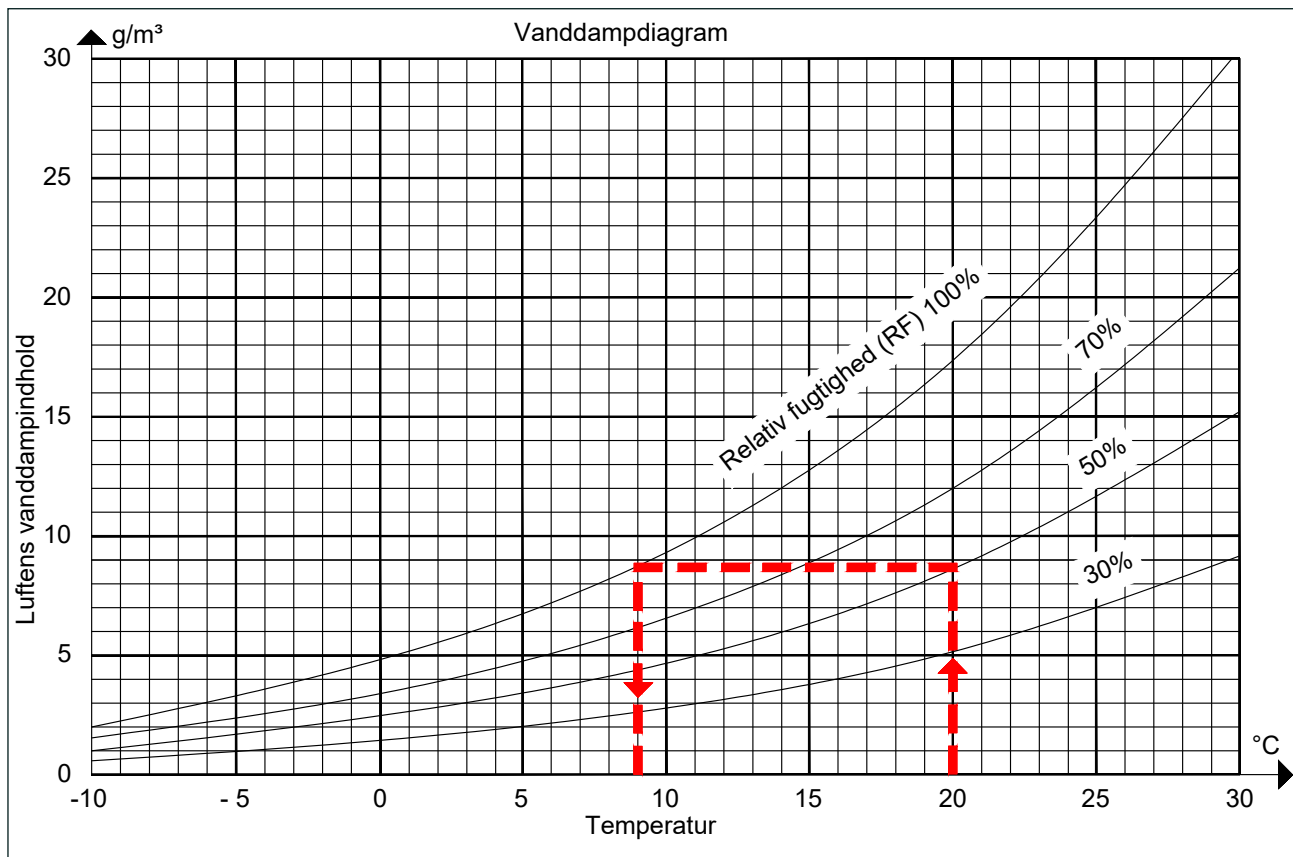
Figur 3.2.1.1: Vanddampdiagram. I det indtegnede eksempel ses, at luften ved en temperatur på 20^{\circ}\text{C} og en relativ luftfugtighed på 50 % RF indeholder ca. 9 g vand pr. \text{m}^3 . Denne lufts dugpunkt er ca. 9^{\circ}\text{C} .
