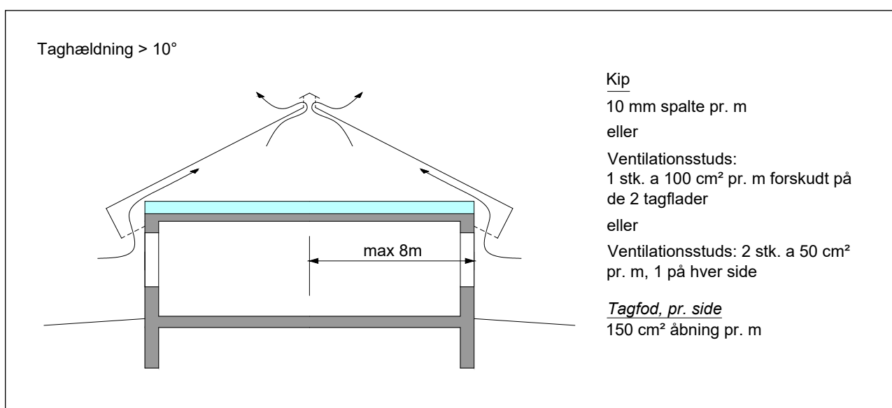
Figur 3.6.1.6: Nettoareal af ventilationsåbninger ved ventilation fra tagfod til dobbeltkip ved taghældning > 10°.
