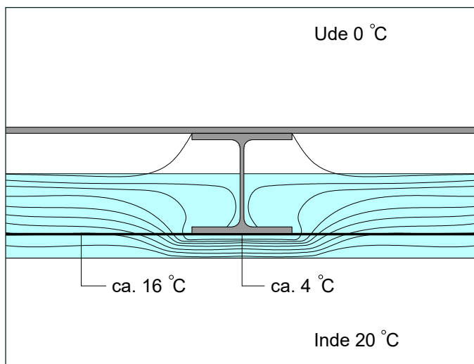
Figur 3.2.3.3: Simulering af temperatur i tagkonstruktion med bærende I-profil af stål. Overfladetemperatur på dampspærre er ca. 16 °C og ca. 4 °C ud for kuldebroen ved stålprofilet, hvilket vil give kondens.
