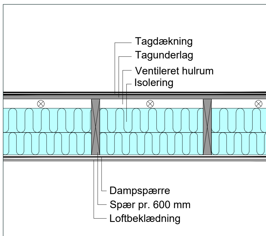
Figur 3.6.1: Ventileret bjælkespærkonstruktion.
