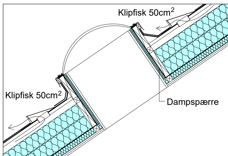
Figur 3.6.5.2: Udskramning eller klipfisk ved tage med hældning over 10°.
