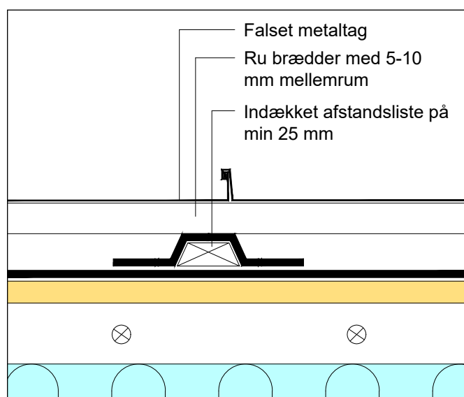
Figur 11.2.3 Falset metaltag udlagt på bræddeunderlag over fast undertag med inddækkede afstandslister.
