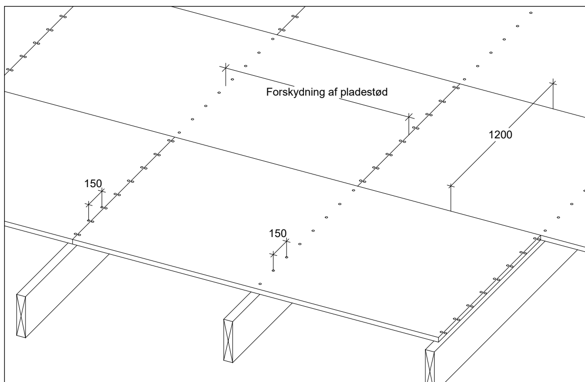
Figur 3.2.1.1 Oplægningssmønster for 15 mm krydsfinerplader med pladedimension 2,44 x 1,22 m
