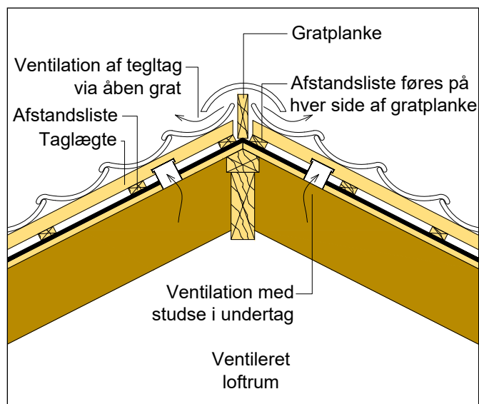
Figur 12.3.1.1 Grat på tag med mørtelfri rygning - vandret snit. Bemærk, at der skal føres afstandslistes på hver side af gratplanken. Ventilation (her vist med studse) monteres i underlag mellem hvert spærfag i gratkonstruktionen. Ventilationen af undertaget kan også udføres med "fisk", som vist på figur 12.2.2.1.
