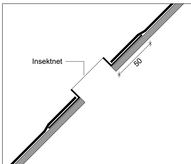
Figur 4.1 Ventilationsstuds med flange til klæbning af tagpap
