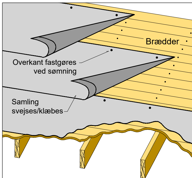
Figur 7.1.1.2 Tagpapbaner kan også fastgøres vinkelret på tagets faldretning
