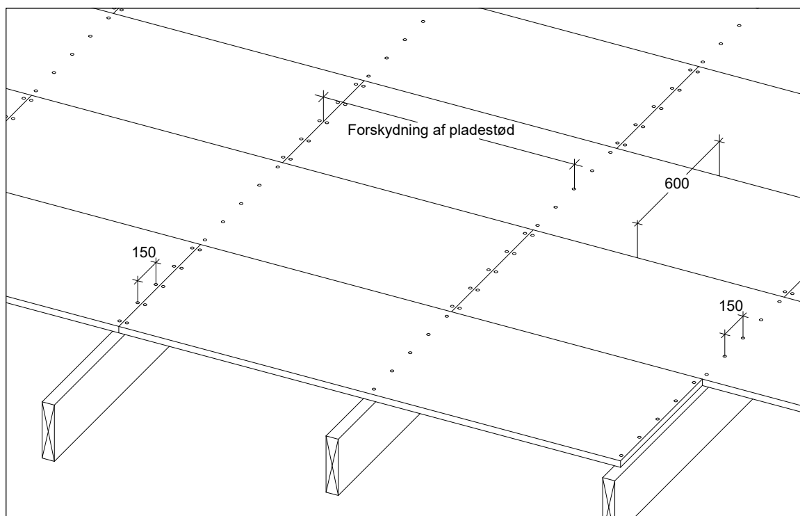
Figur 3.2.1.2 Oplægningssmønster for 15 mm krydsfinerplader med pladedimension 0,61 x 2,44 m
