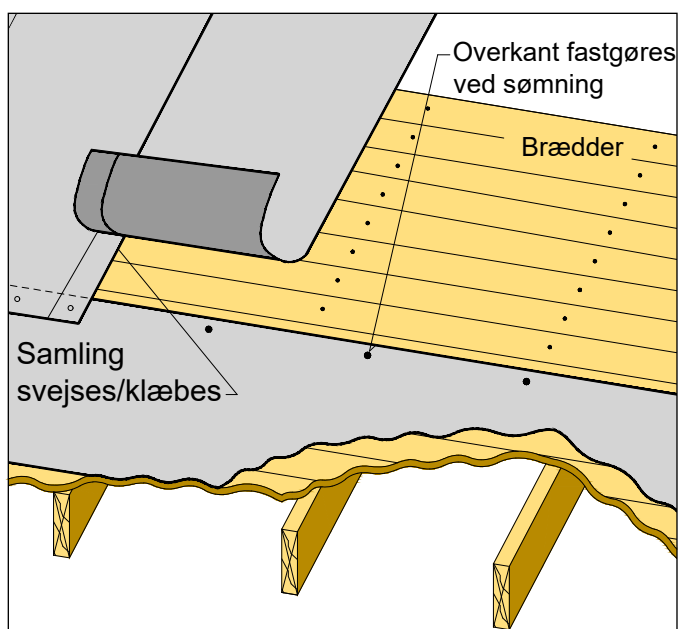
Figur 7.1.1.1 Tagpapbaner sømmes til bræddeunderlag (eller plader) parallelt med eller vinkelret på tagets faldretning. Fastgørelse til underlaget sker pr. 150-200 mm og 2 cm fra kanten. For at forhindre at vindsug under byggeperioden river tagpappen løs, monteres afstandslisters i takt med udlægning af tagpap
