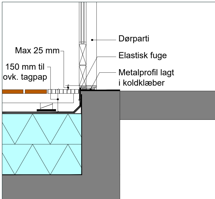
Figur 2.4.3.3.: Niveaufri adgang – tremmegulv af træ. Højdeforskellen mellem terrassebelægning og toppen af dørens bundstykke må højest være 25 mm (se SBI-anvisning 222).
