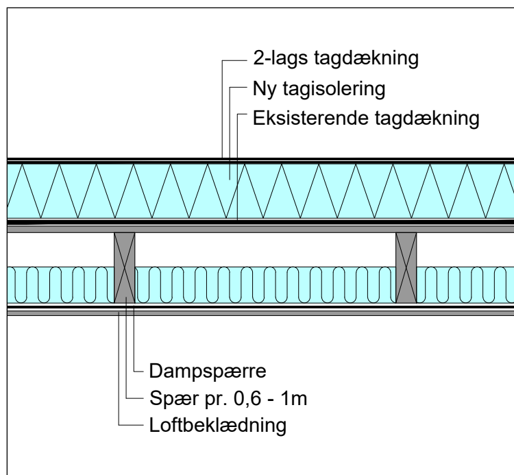
Figur 3.2.1.1: Renovering med udvendig merisolering på koldt tag. Tykkelse af merisoleringslaget afhænger af fugtbelastningen. Se PTM-anvisning 4. Fugt.
