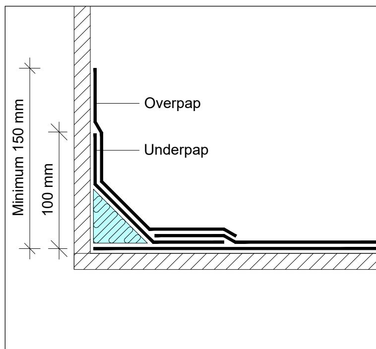
Figur 3.3.1.1: Princip for inddækning af 2-lags tagdækning mod lodret kant.
